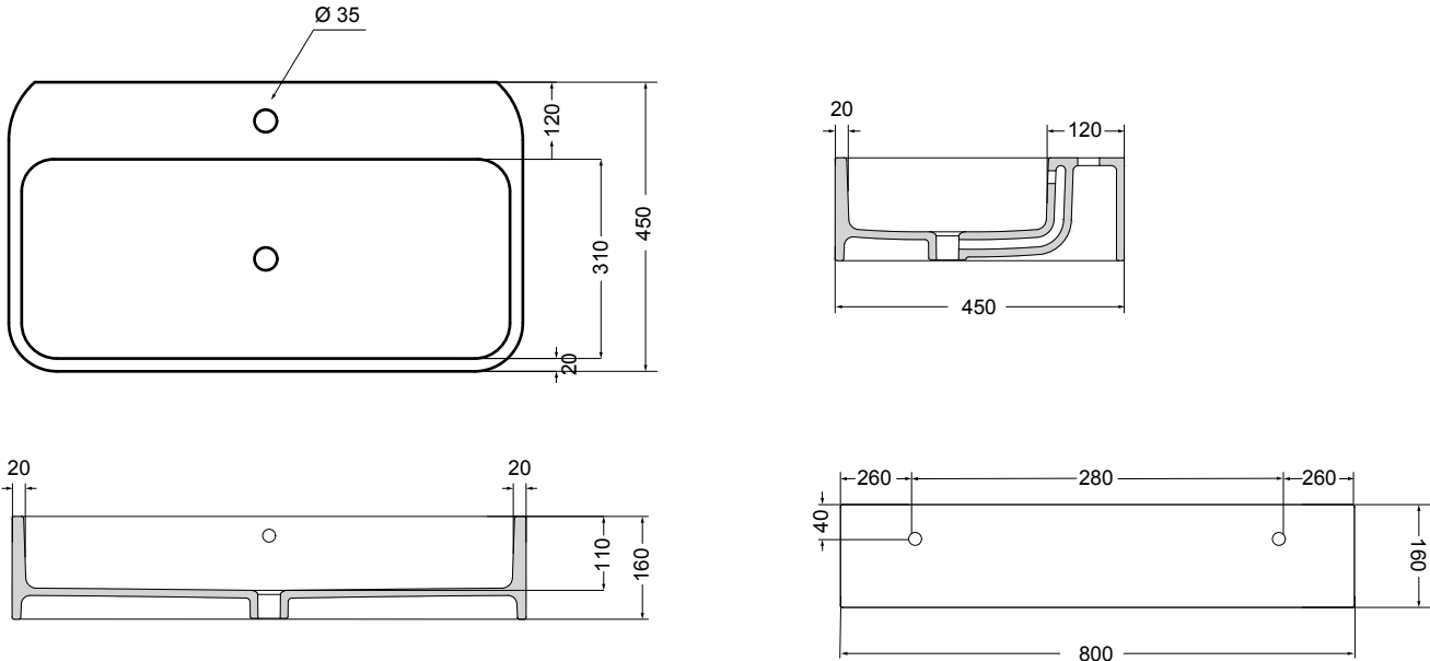
86300 lavabo appoggio/sospeso 80x45 cm_counter-top/wall-hung basin 80x45 cm
