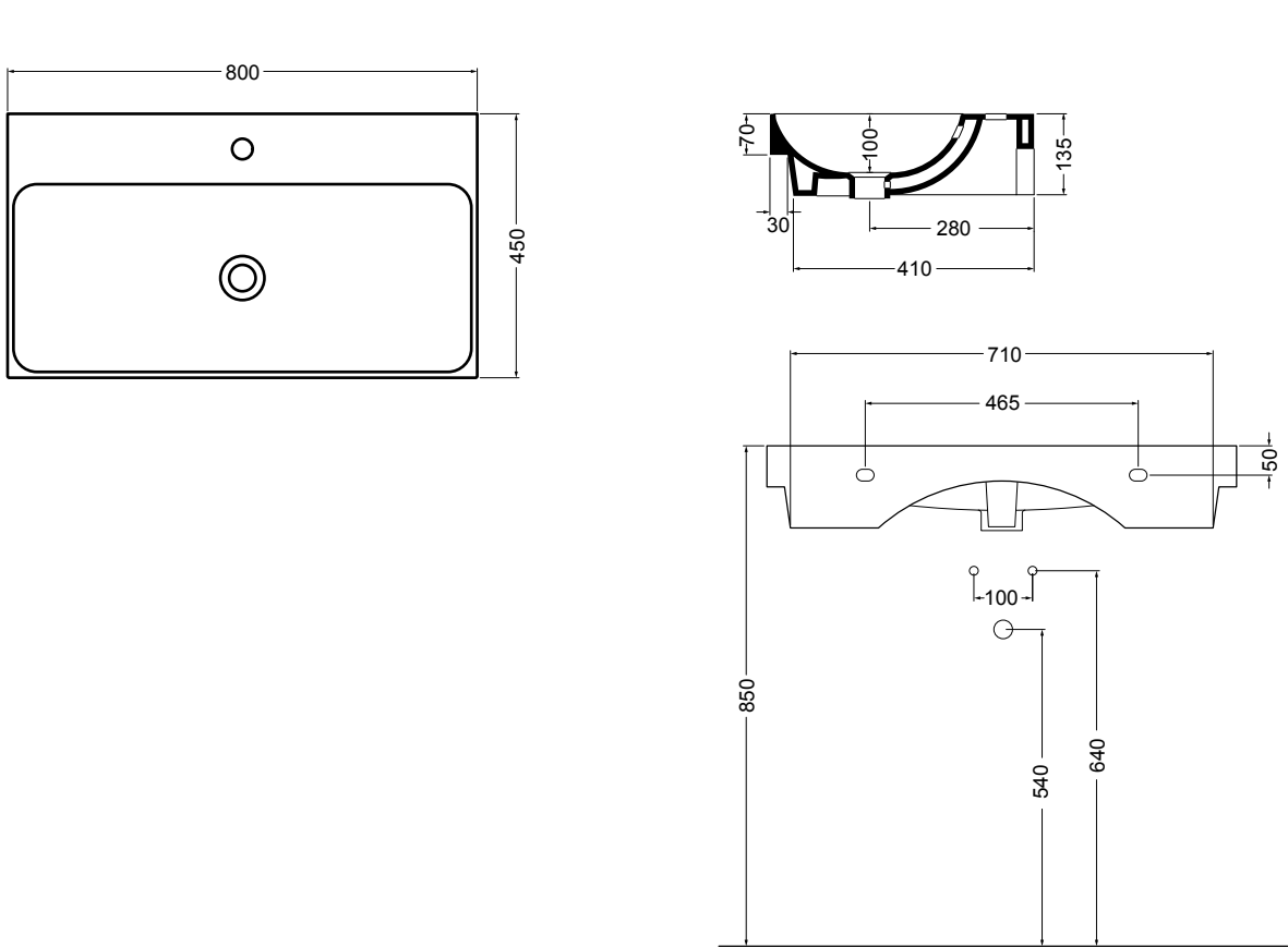
WS110 NORMAL lavabo sospeso, incasso e da appoggio 80 cm_NORMAL wall hung, inset and counter-top basin 80 cm
