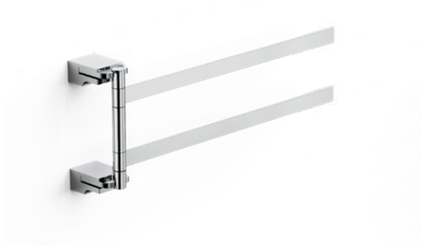
SW111 - interasse / ctc distance 10,4 cm
