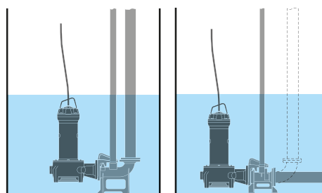
Installazione con DISPOSITIVO DI ACCOPPIAMENTO DA FONDO
