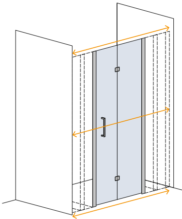
PORTA DOPPIO BATTENTE "SU MISURA"
