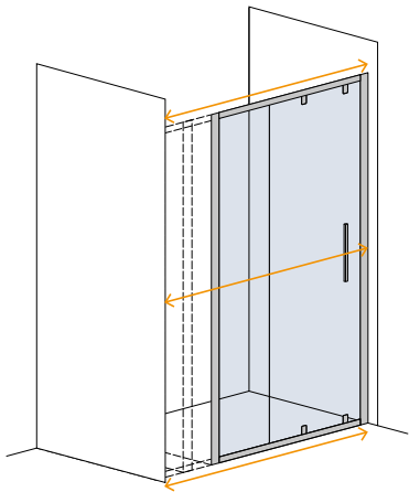
PORTA DOPPIO SCORREVOLE "SU MISURA"
