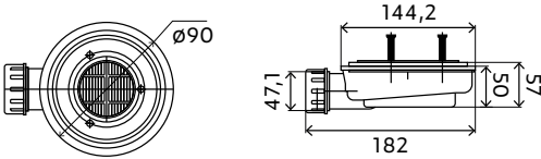
PILETTA DI SCARICO PIATTO DOCCIA
