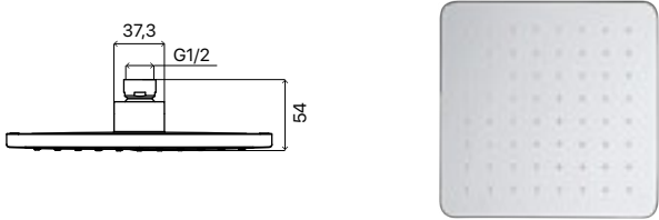
Soffione Abs quadro.
