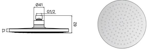
Soffione Abs tondo.
