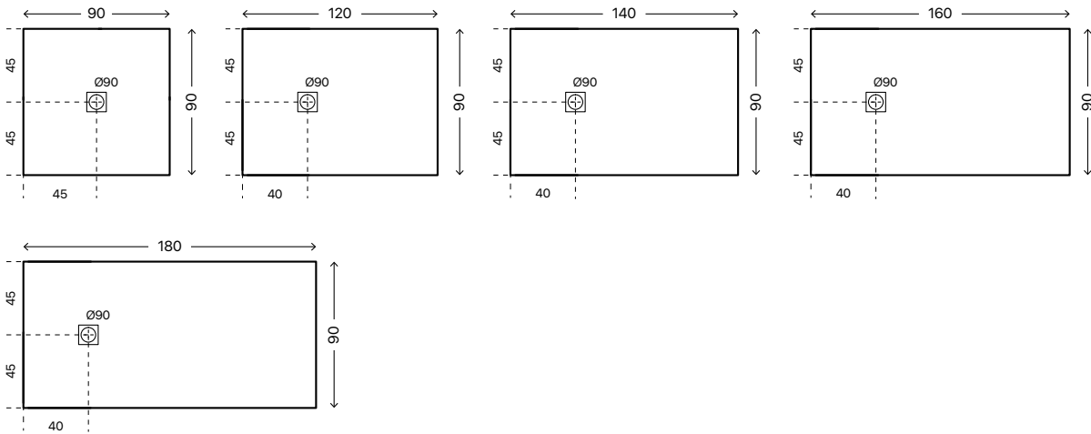
PILETTA DI SCARICO PIATTO DOCCIA
