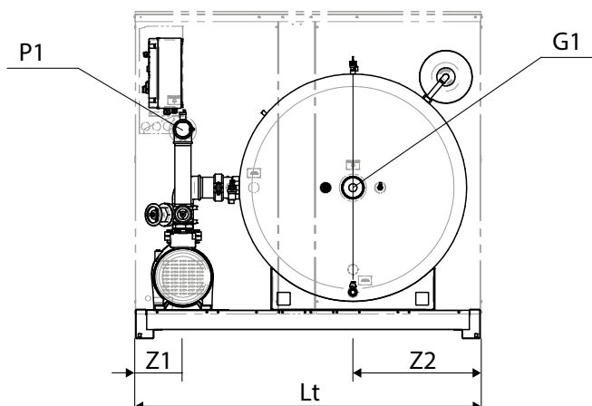
Dimensioni HPT orizzontali
