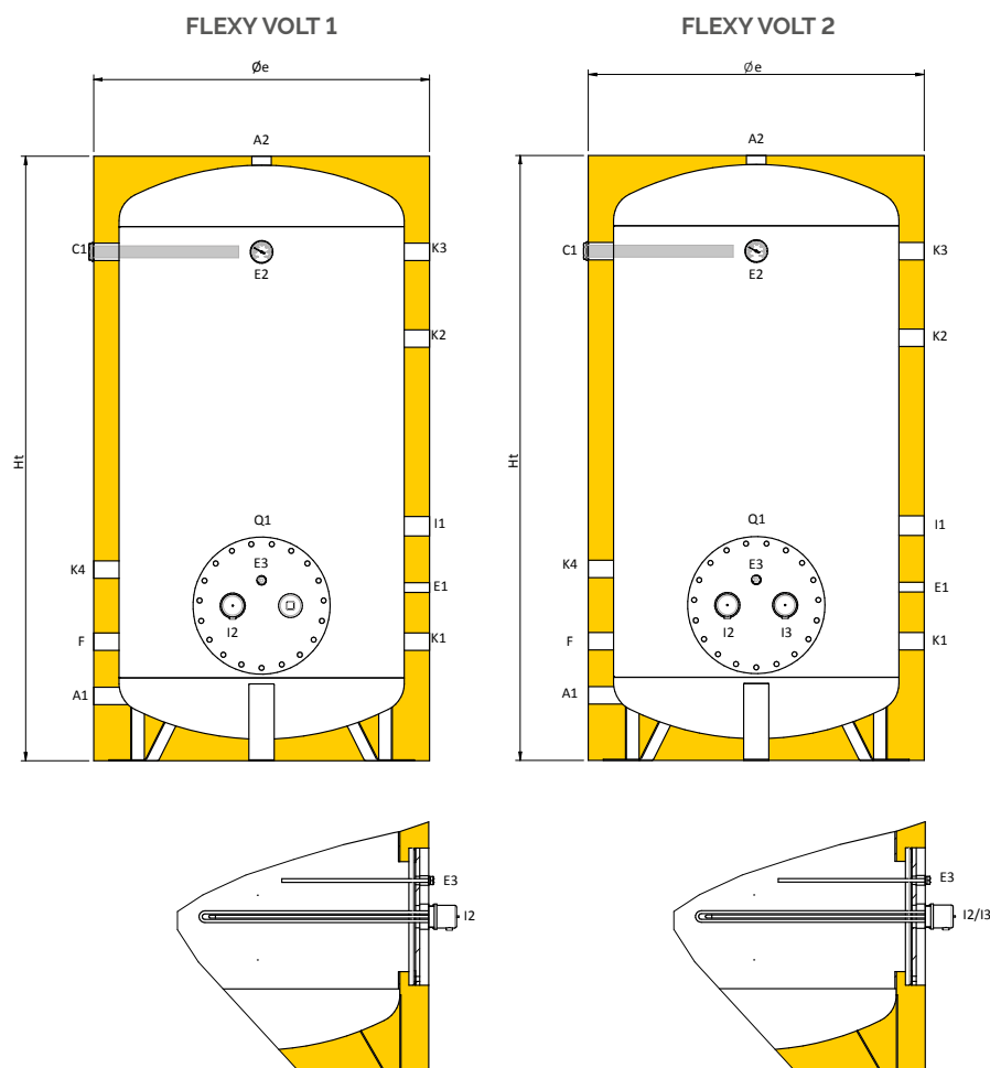
Legenda connessioni
