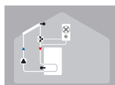
Solare con raffreddamento 1 (raffreddamento collettore)
