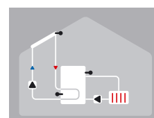
Solare con raffreddamento 3 (raffreddamento collettore)
