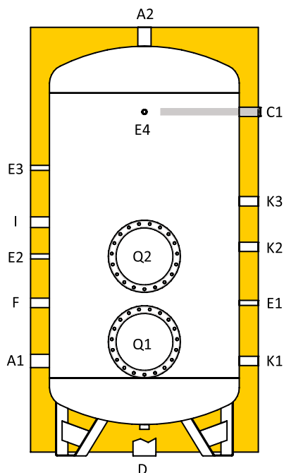
Legenda connessioni
