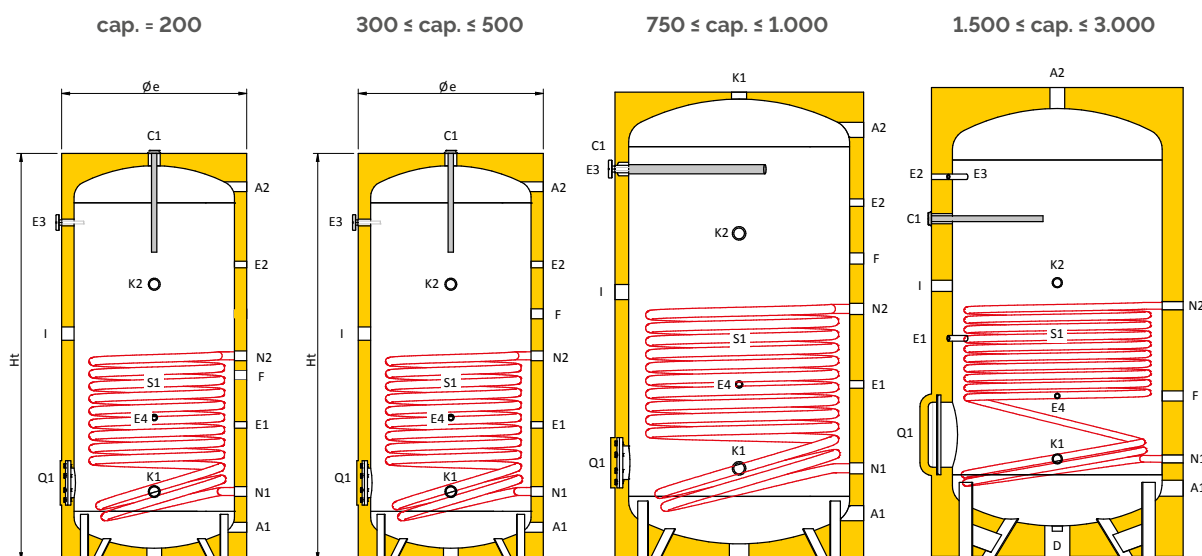
Legenda connessioni
