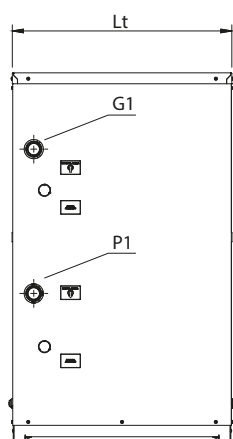
Dimensioni HPT verticali
