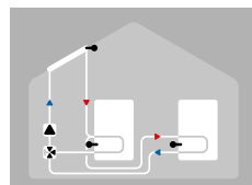
Solare con 2 accumuli e valvola
