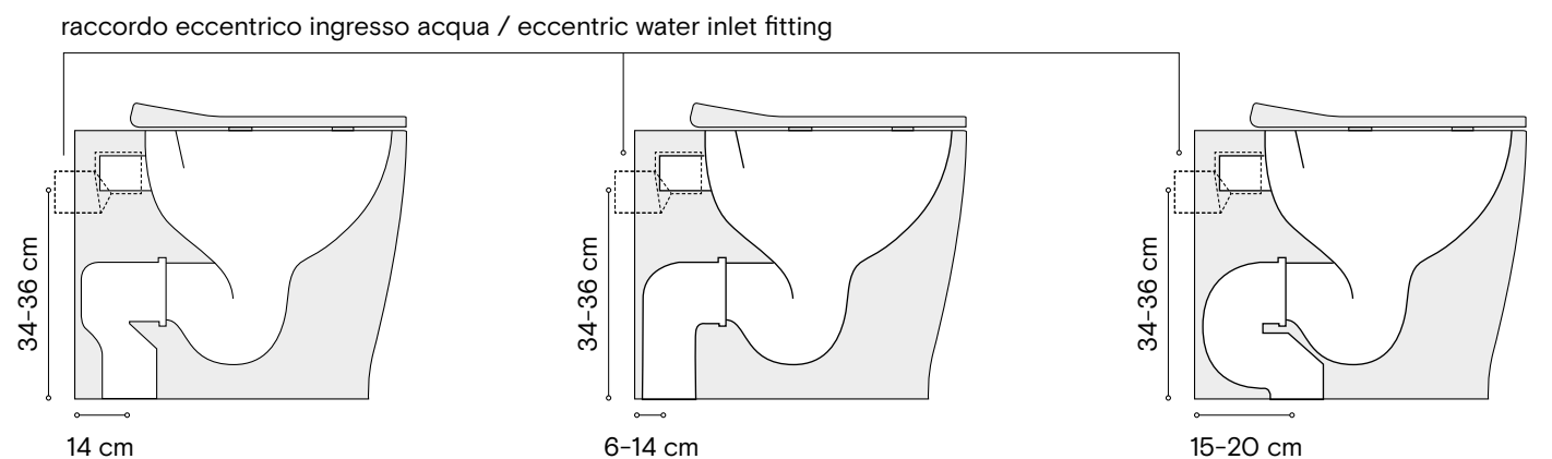
CURVA TECNICA SCARICO FISSO 14 CM / TECHNICAL CURVE FIXED DRAIN 14 CM
