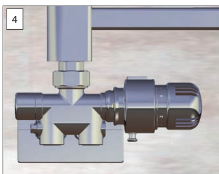
4 Installare il comando sulla valvola facendo combaciare gli incastri
