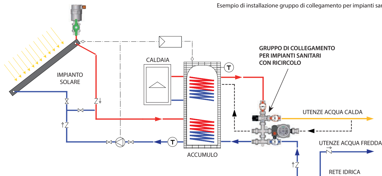
Esempio di installazione gruppo di collegamento per impianti sanitari
