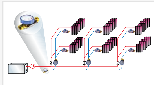
Fig.2 - Impianto bilanciato
