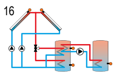
Sistema con collettori est/ovest e scambio termico
