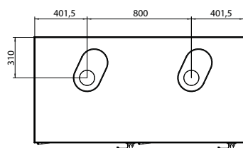
Luna MP 1.35 - 1.50 - 1.60 - 1.70
