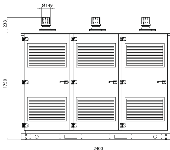
vista frontale
