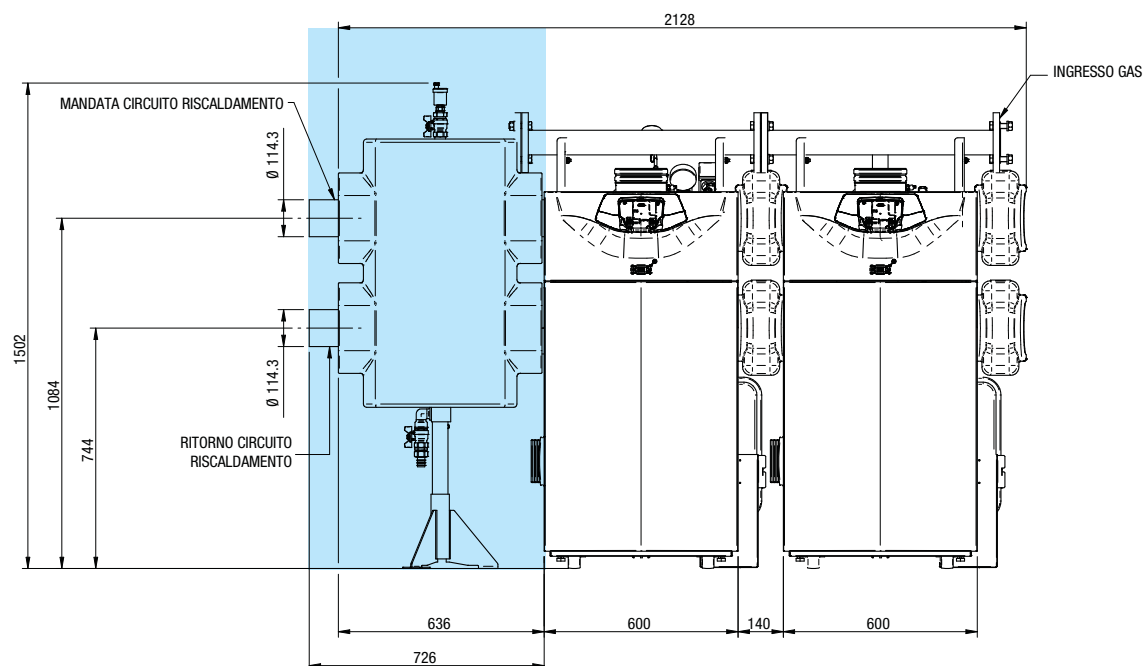
Centrale termica con separatore idraulico
