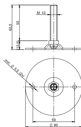
Kit regolazione altezza del telaio cod. A111807
