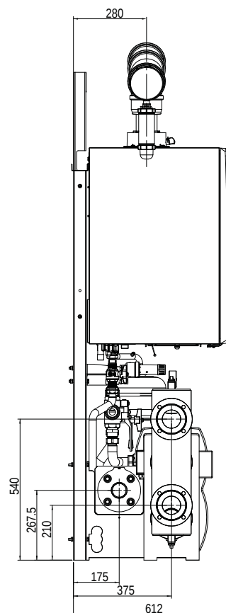
Centrale termica con scambiatore a piastre
