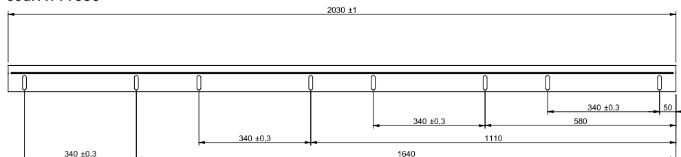
Kit staffe a parete per 4 caldaie cod. A111690
