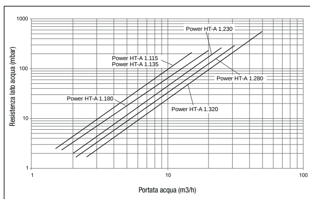
Power HT-A 1.115 - 1.320 Perdite di carico scambiatori
