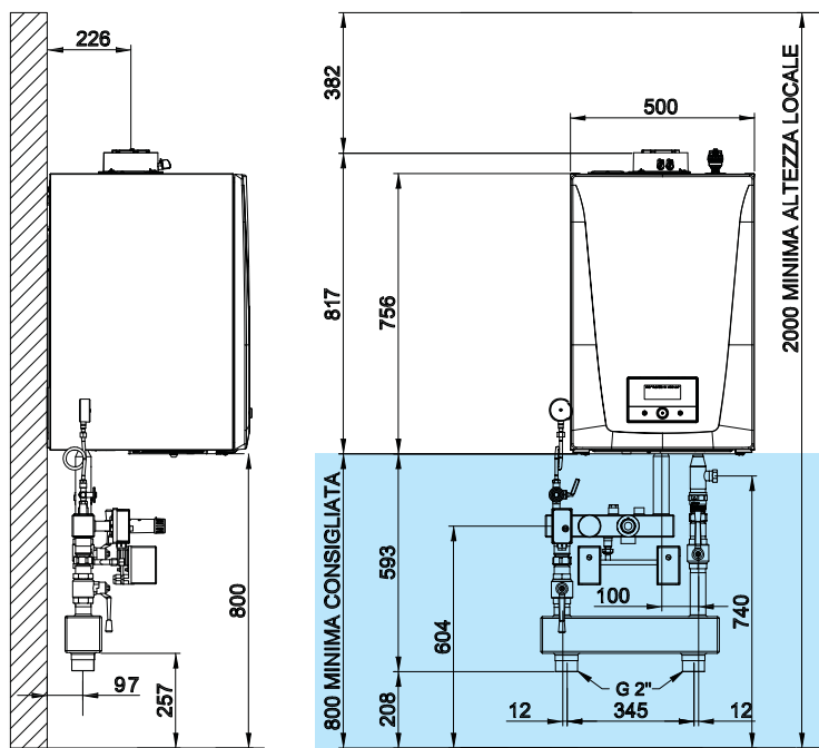
Centrale termica con separatore idraulico
