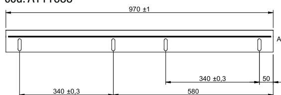
Kit staffe a parete per 2 caldaie cod. A111688
