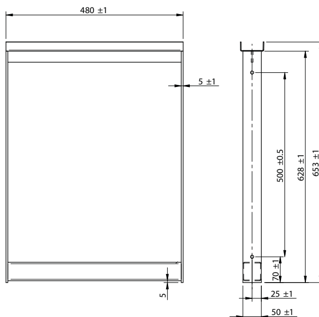
Kit supporto orizzontale per telaio cod. A120918
