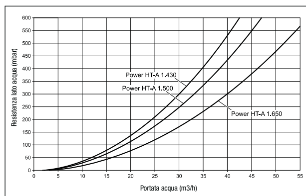
Power HT-A 1.430 - 1.650 Perdite di carico scambiatori
