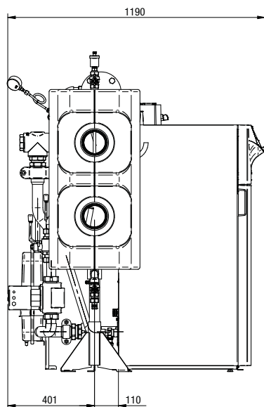
Centrale termica con separatore idraulico
