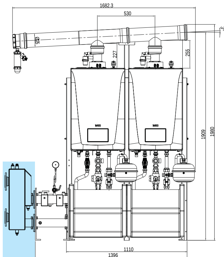
Centrale termica con separatore idraulico
