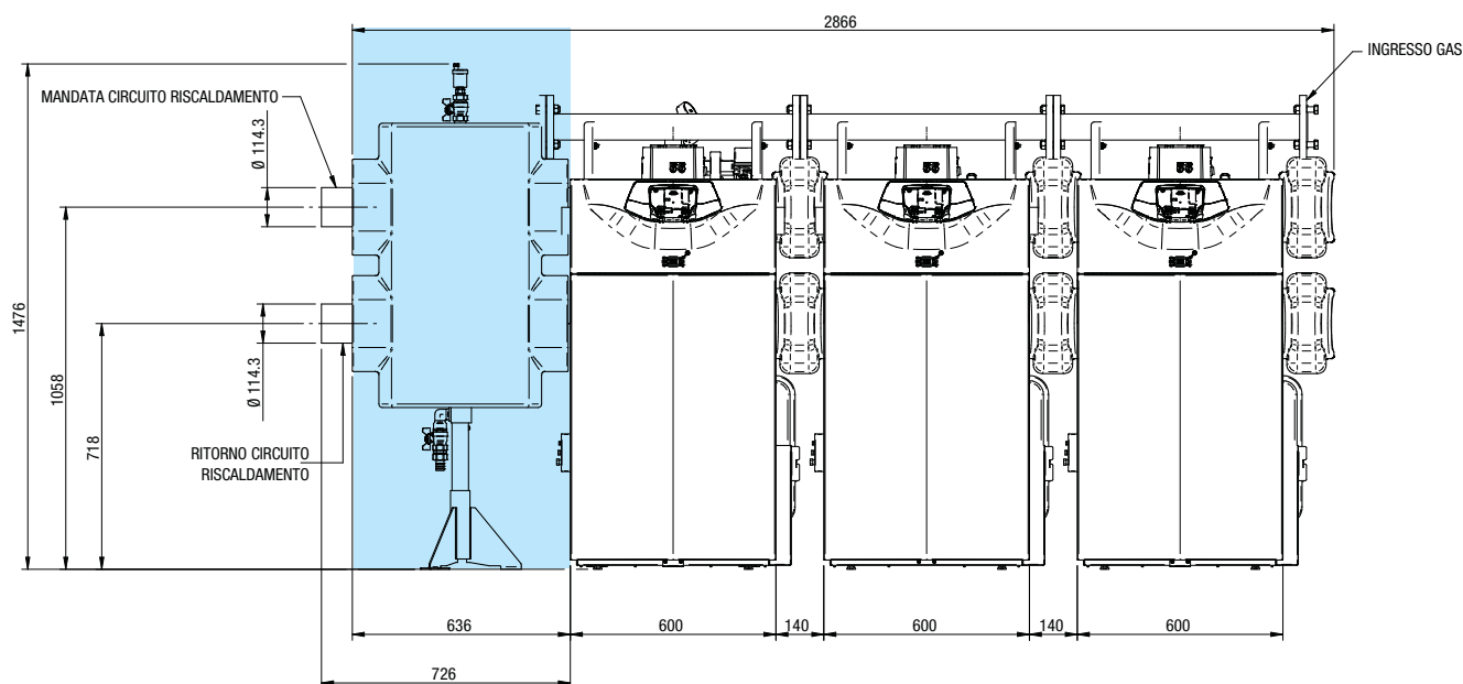
Centrale termica con separatore idraulico
