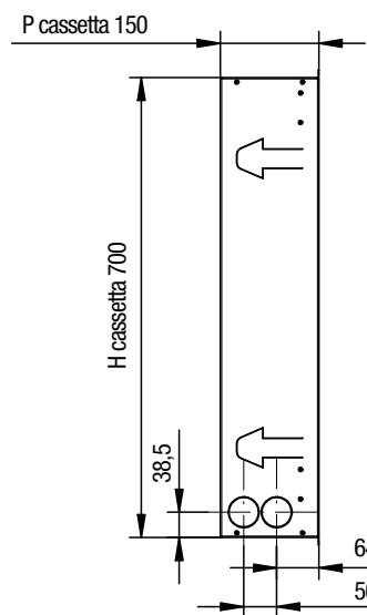
vista laterale da sinistra
