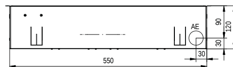
vista dal basso
