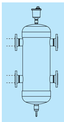
Centrale termica con separatore idraulico
