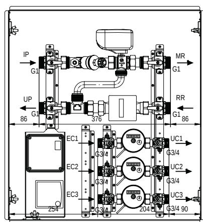
vista frontale
