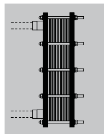
Centrale termica con scambiatore a piastre
