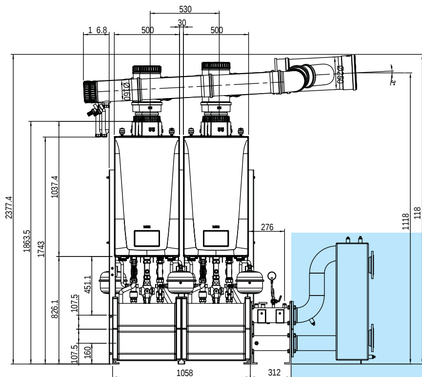
Centrale termica con separatore idraulico
