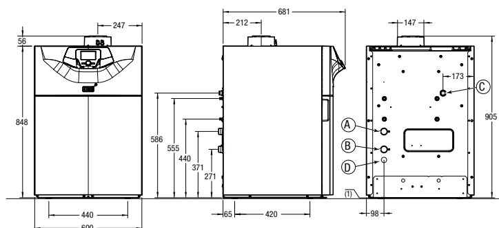
Attacchi idraulici Power HT+ 1.50-1.70
