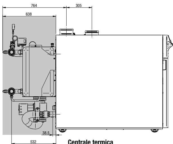
Centrale termica con scambiatore a piastre
