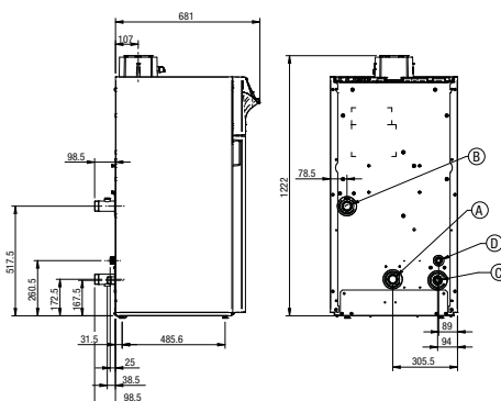
Attacchi idraulici Power HT+ 1.130-1.150
