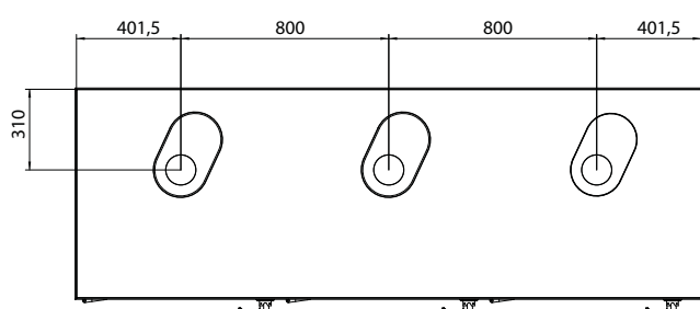
Luna MP 1.35 - 1.50 - 1.60 - 1.70
