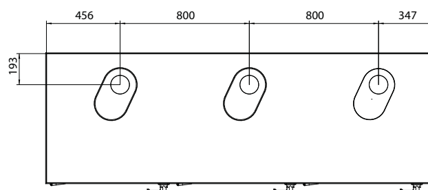
Luna MP 1.90 - 1.110 - 1.115 - 1.130 - 1.150
