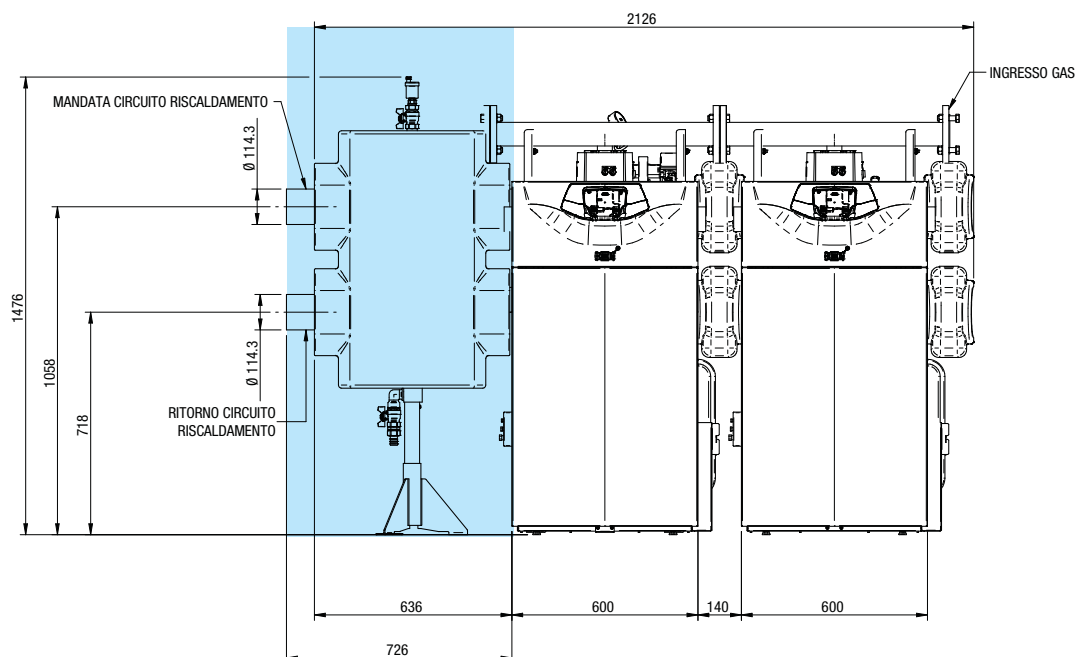
Centrale termica con separatore idraulico
