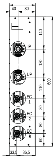
vista da dx
