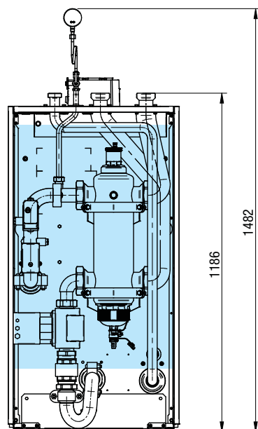
Centrale termica con separatore idraulico
