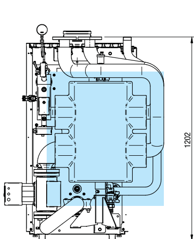
Centrale termica con separatore idraulico
