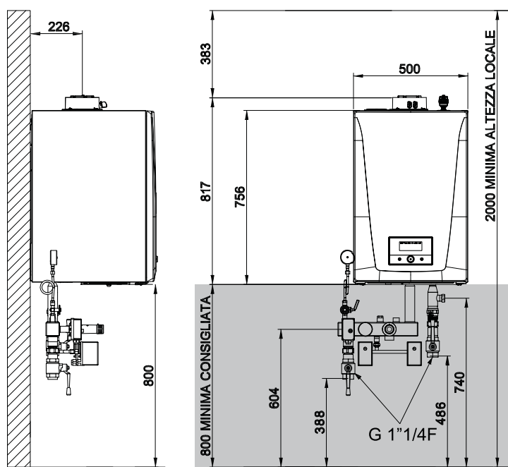
Centrale termica con scambiatore a piastre
