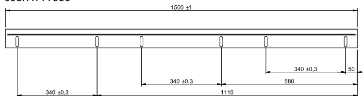
Kit staffe a parete per 3 caldaie cod. A111689
