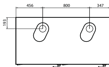
Luna MP 1.90 - 1.110 - 1.115 - 1.130 - 1.150
