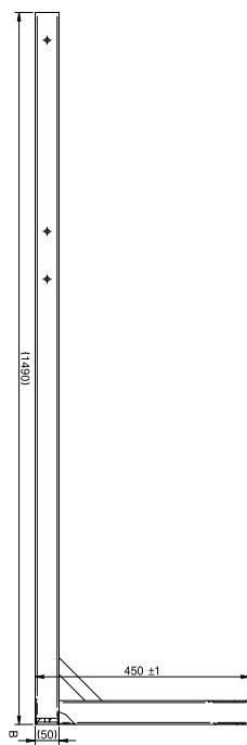
Kit supporto verticale a L per telaio cod. A7866380
