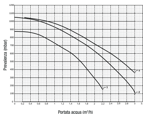
CURVA PORTATA PREVALENZA POMPA ALLA PLACCA Luna MP 1.35 - 1.50 - 1.60 - 1.70
