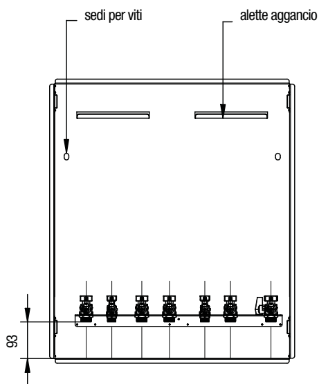
vista frontale
