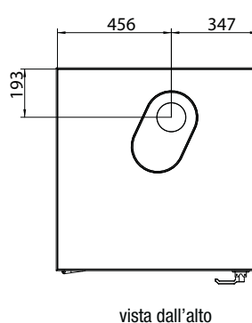
Luna MP 90-110
