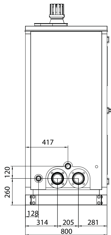
vista laterale
