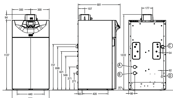
Attacchi idraulici Power HT+ 1.90-1.110
