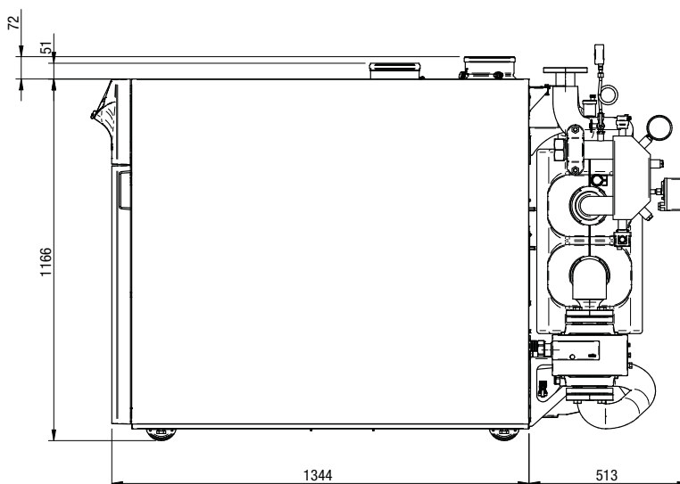
Ø collettori mandata/ritorno DN50 Ø collettore gas G 1 ½ "
