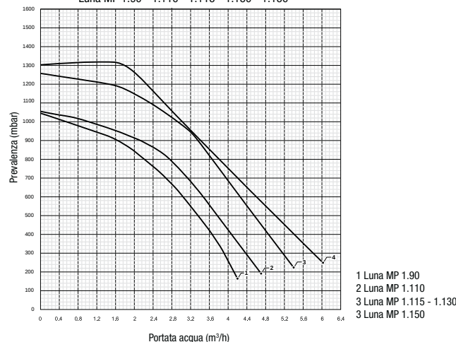
CURVA PORTATA PREVALENZA POMPA ALLA PLACCA Luna MP 1.90 - 1.110 - 1.115 - 1.130 - 1.150
