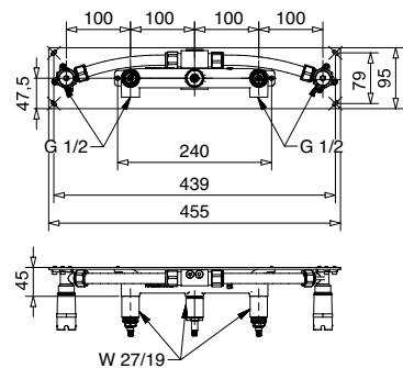
19889 Blocco incasso per gruppo con bocca e kit duplex Built-in part for mixer with spout and kit duplex
