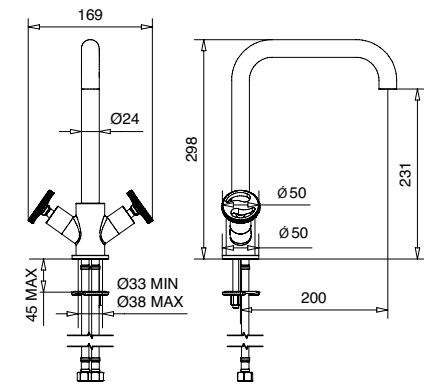
MILLENOVECINQUANTA Monoforo lavello canna tubo girevole con flex inox Single hole sink mixer swivel tube spout with flex
