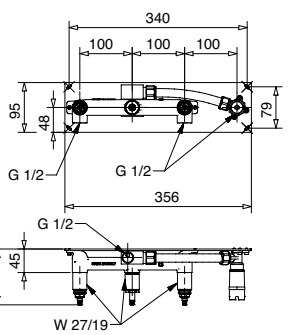
19882 Blocco incasso per gruppo con soffione e kit duplex Built-in part for mixer with big shower and kit duplex
