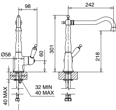
OXFORD Monocomando monoforo lavello piantone alto canna girevole con flex inox Single hole sink mixer high swivel spout with flex inox
