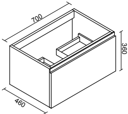
Base sospesa porta lavabo con 1 cassetto Wall wash-stand with 1 drawer
