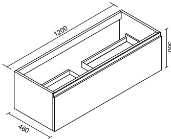
Base sospesa porta lavabo con 1 cassetto Wall wash-stand with 1 drawer
