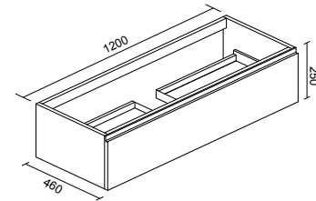
Base sospesa porta lavabo con 1 cassetto Wall wash-stand with 1 drawer
