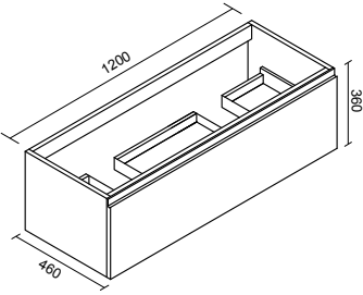
Base sospesa porta lavabo doppia vasca con 1 cassetto Double sink wall wash-stand with 1 drawer
