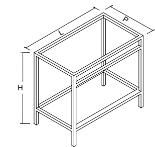
Kit struttura Structure kit
