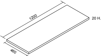
Top superiore di chiusura base Close-up top for cabinet
