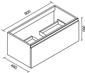
Base sospesa porta lavabo con 1 cassetto Wall wash-stand with 1 drawer
