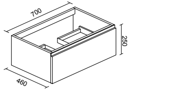
Base sospesa porta lavabo con 1 cassetto Wall wash-stand with 1 drawer
