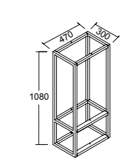
Kit struttura Structure kit
