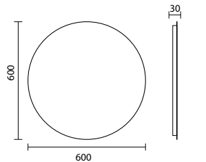
Specchiera circolare LED retroilluminata senza cornice Circular LED blacklit mirror without frame
