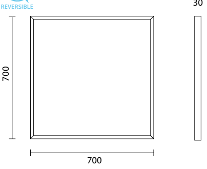
Specchiera con cornice nera Black mirror with frame
