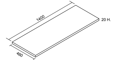
Top superiore di chiusura base Close-up top for cabinet
