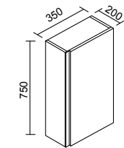
Pensile sospesa con 1 anta Wall unit cabinet with 1 door
