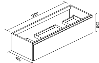
Base sospesa porta lavabo doppia vasca con 1 cassetto Double sink wall wash-stand with 1 drawer
