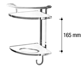
603 Angolare doccia Shower corner tray L. 180 H. 315 P. 195 mm
