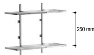
C452 Scaffale 2 piani 2-level shelf unit L. 450 H. 380 P. 162 mm
