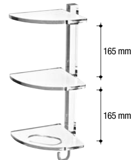
606 Angolare doccia Shower corner tray L. 160 H. 450 P. 180 mm
