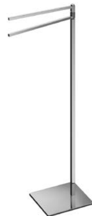
C474/M574 Piantana lavabo Washbasin stand L. 390 H. 840 P. 200 mm Base 220 x 180 mm
