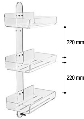
1223 - 1233 Portaoggetti Accessory holder 1223 - L. 200 H. 630 P. 155 mm 1233 - L. 300 H. 630 P. 155 mm
