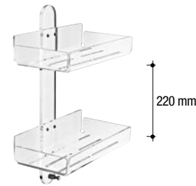
1222 - 1232 Portaoggetti Accessory holder 1222 - L. 200 H. 430 P. 155 mm 1232 - L. 300 H. 430 P. 155 mm
