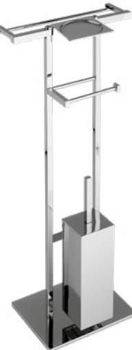
3075 Piantana wc-bidet Toilet-bidet stand Base 220x180 L. 280 H. 760 mm
