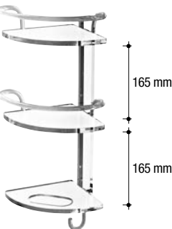
604 Angolare doccia Shower corner tray L. 180 H. 490 P. 195 mm
