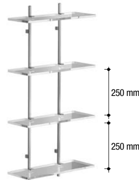
C454 Scaffale 4 piani 4-level shelf unit L. 450 H. 900 P. 162 mm
